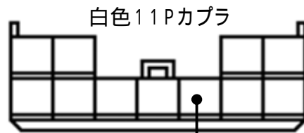
ドアスイッチ配線(茶色線)
