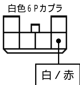
L端子配線(灰色線)
