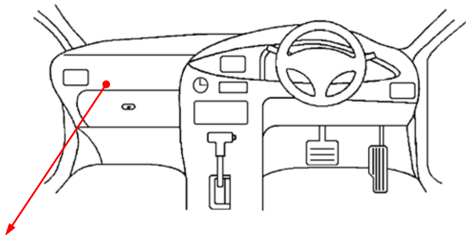
ドアスイッチ配線(茶色線)
