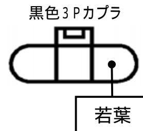
L端子配線(灰色線) (オルタネーター直)
