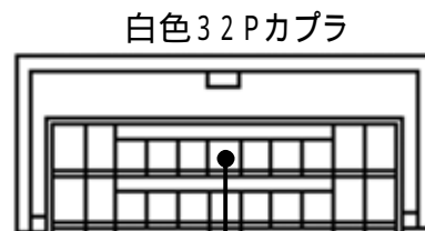
L端子配線(灰色線)
