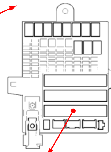
ドアスイッチ配線(茶色線)
