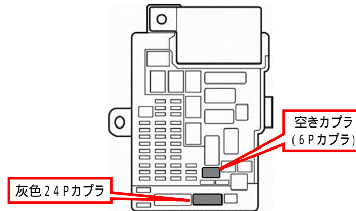
ヒューズブロック表側
