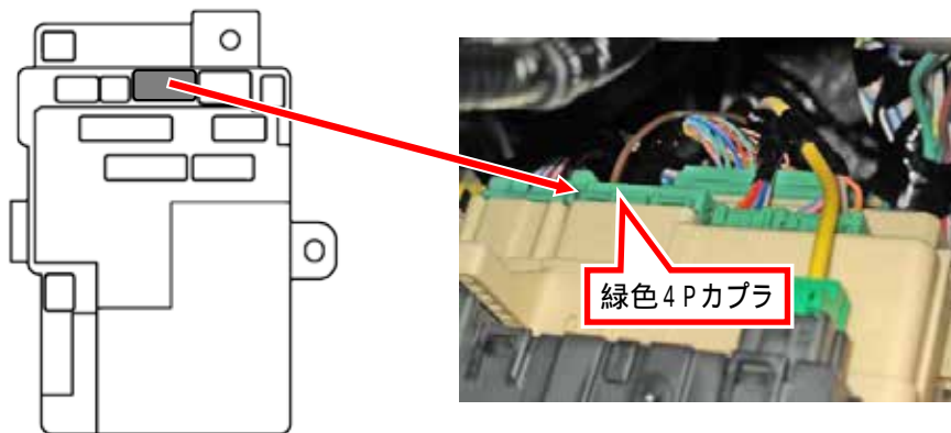
ヒューズブロック裏側
