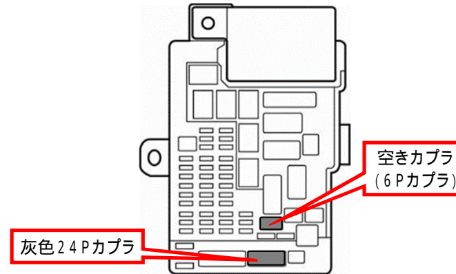
ヒューズブロック表側
