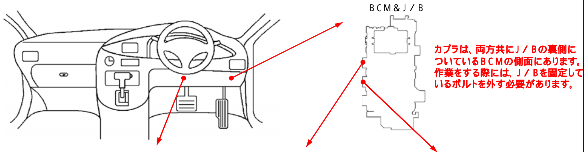
フットブレーキ配線(白色線)
