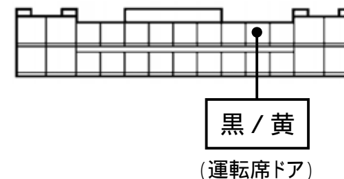
灰色26Pカプラ
