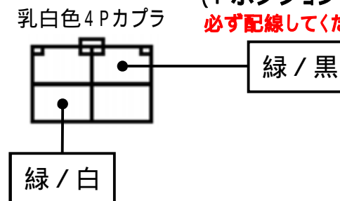
フットブレーキ配線(白色線)
