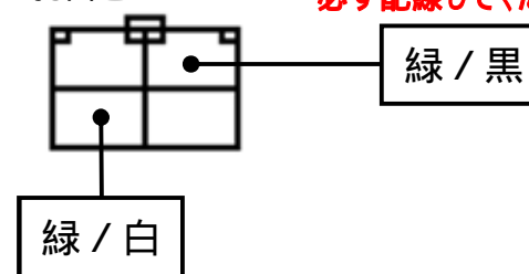
フットブレーキ配線(白色線)
