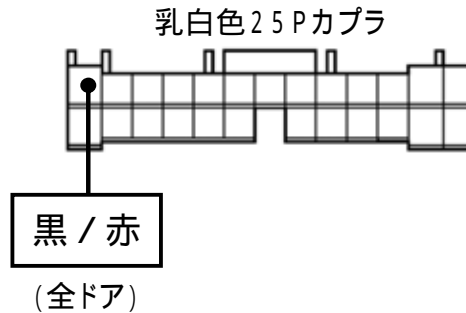
ドアスイッチ配線(茶色線)
