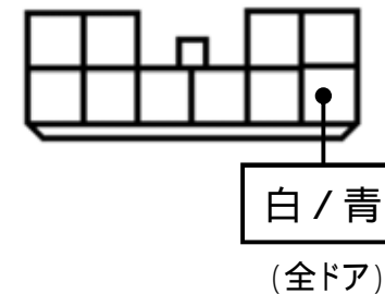
白色10Pカプラ
