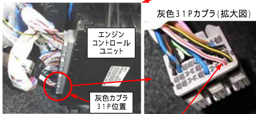
白 / 赤線へ接続
