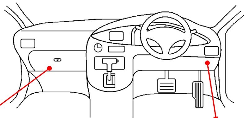
イモビアダプター「IM84」 IM84専用ハーネス 2Pコネクタの接続
