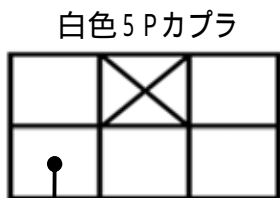
L端子配線(灰色線)
