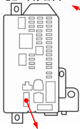
ドアスイッチ配線(茶色線)
