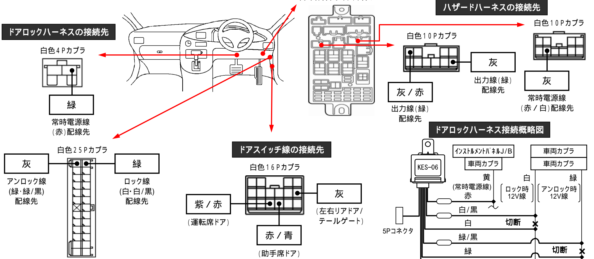
インストルメントパネルJ/B
