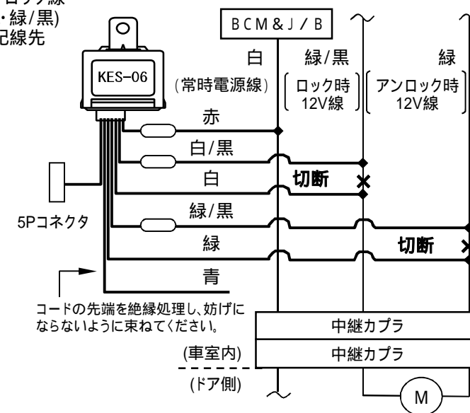
ドアロックハーネス接続概略図
