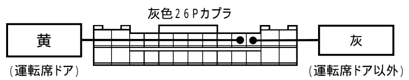
ドアスイッチ線の接続先
