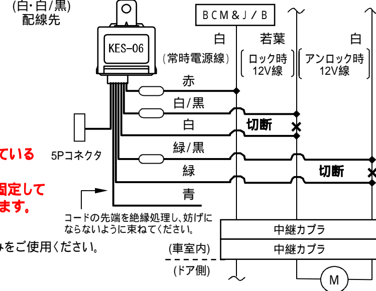
ドアロックハーネス接続概略図
