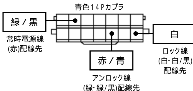
ドアロックハーネスの接続先
