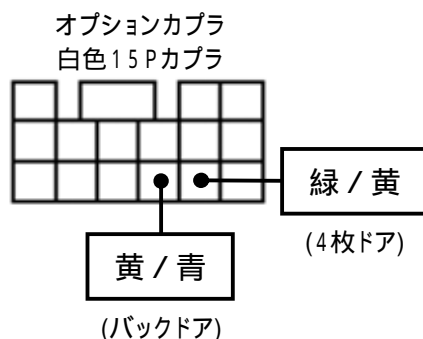
ドアスイッチ線の接続先
