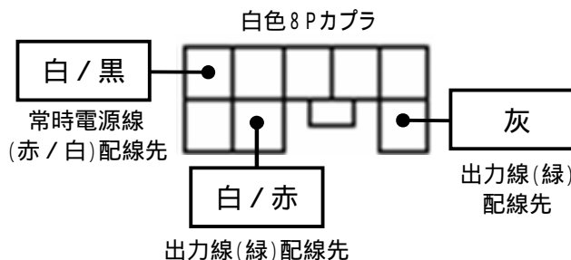
ハザードハーネスの接続先
