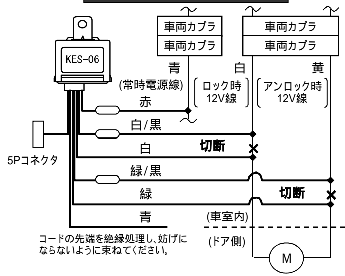
ドアロックハーネス接続概略図
