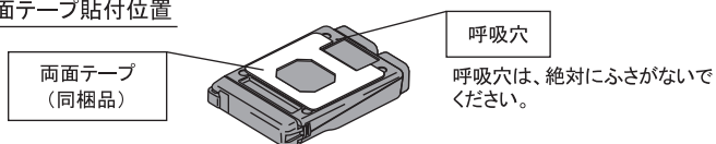
両面テープ貼付位置
