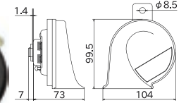
寸法図
