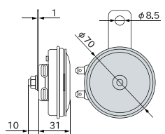
寸法図
