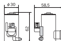
寸法図
