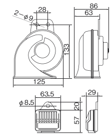
寸法図
