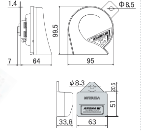
寸法図
