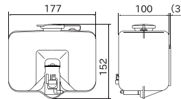
寸法図
