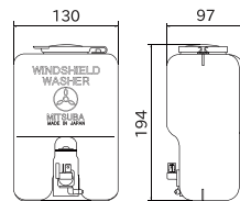
寸法図
