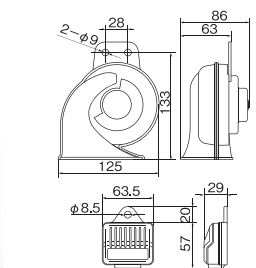
寸法図
